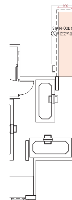
Tower 6 Upper Roof Part Plan 第6座 上層天台 局部平面圖
